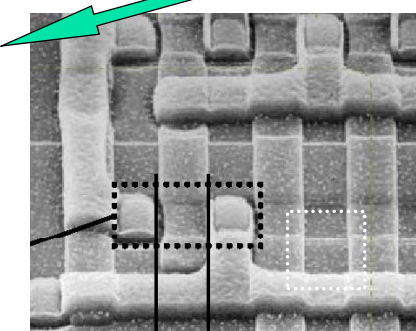
Del av overflaten forstørret – 1 transistor, 0.0001 mm linjebredde ( 100nm)
