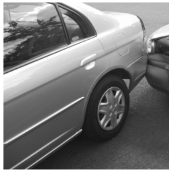
Gråtonebilde
