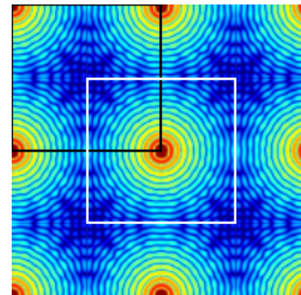
|F(u,v)| : Fourier-spekteret
