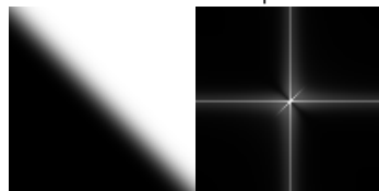
Bilde Fourier-spekter
