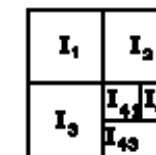
(d) Merge
