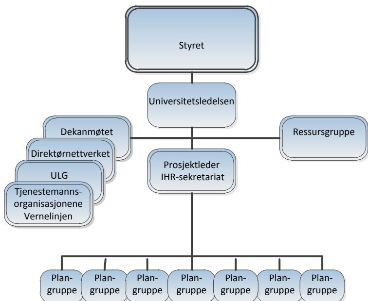
Figur 4: Prosjektorganisasjon
