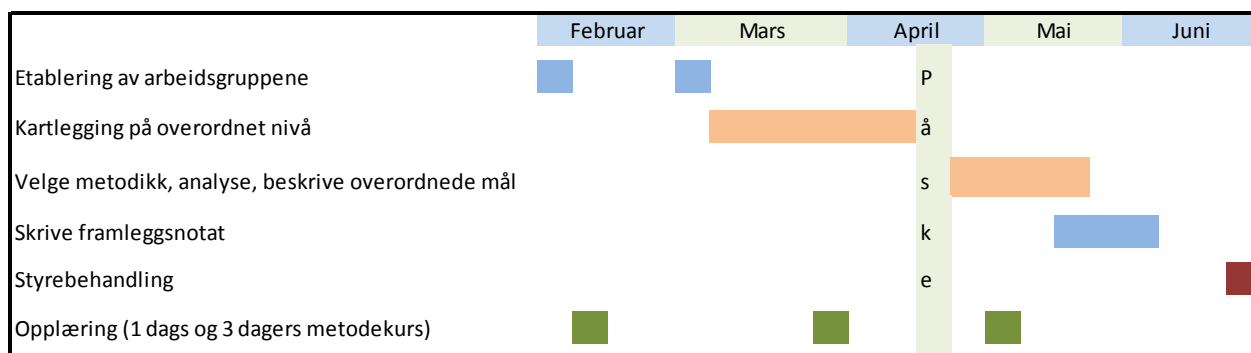
Fig 5: Overordnet fremdriftsplan
