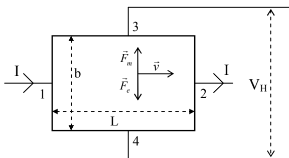
Fig.1: Halvlederkristall med parametre for beregning av Hall-spenningen.
