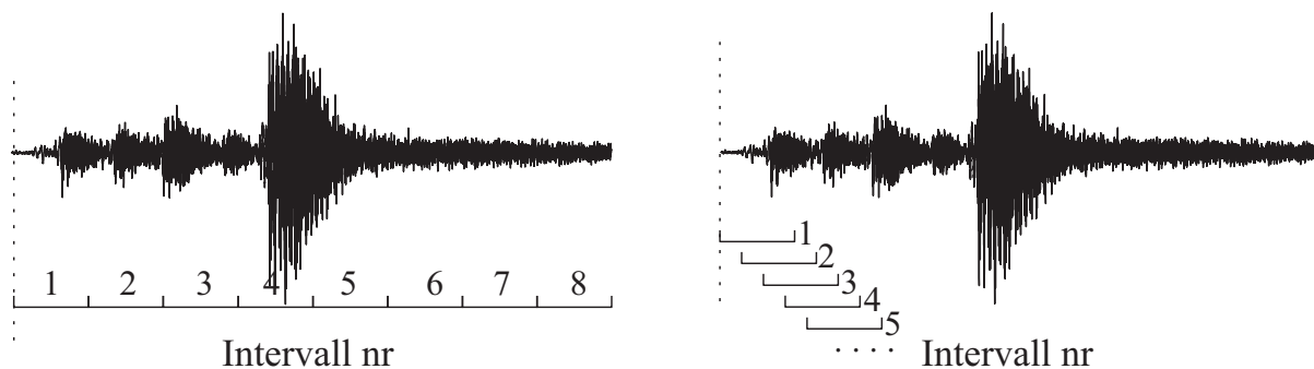
Figur 13.1: For å få tidsinformasjon ved analyse av en lang tidsstreng med data, kan vi stykke opp det totale tidsintervallet og foreta fouriertransformasjon for intervall etter intervall. Intervallene kan velges slik at de ikke overlapper hverandre (venstre del) eller slik at de overlapper hverandre (høyre del). Se teksten for vurdering av disse teknikkene.
