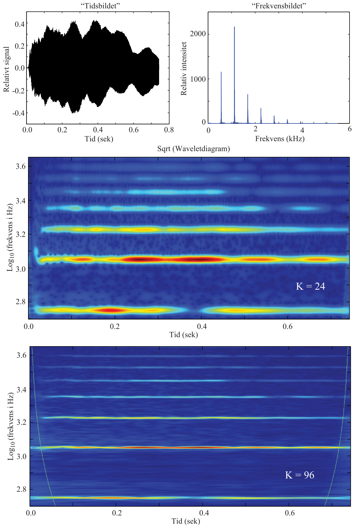
Figur 13.13: En ren trompetlyd analysert i tidsbildet, i frekvensbildet og i en wavelettransformasjon. To ulike K -verdier er brukt i waveletanalysen.
