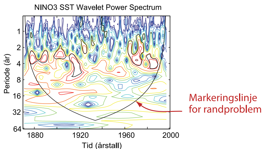
Figur 13.9: Eksempel på et waveletdiagram for temperaturoscillasjoner i det sydlige stillehav. Figuren er produsert med data og programvare tilgjengelig fra http://paos.colorado.edu/research/wavelets/ tilgjengelig april 2013.
