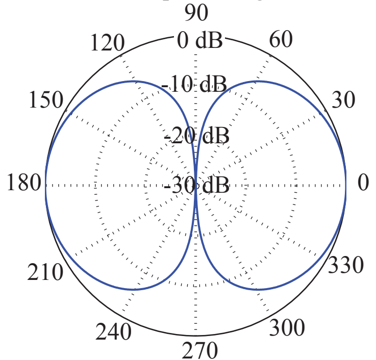
Antennekarakteristikk for en vanlig vertikal dipolantenne. Det er rotasjonssymmetri rundt den vertikale antennen.
