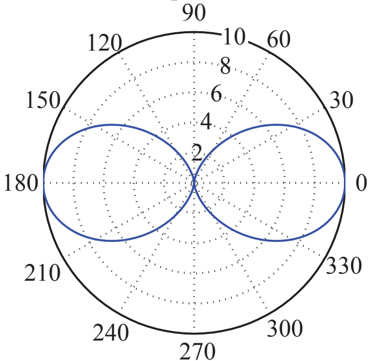
Antennekarakteristikk for en vanlig vertikal dipolantenne. Det er rotasjonssymmetri rundt den vertikale antennen.
