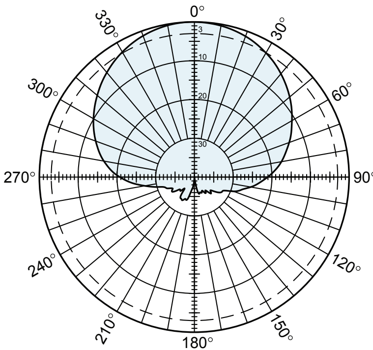
Antennekarakteristikk for en vanlig basestasjonsantenne for GSM900 mobiltelefoni
