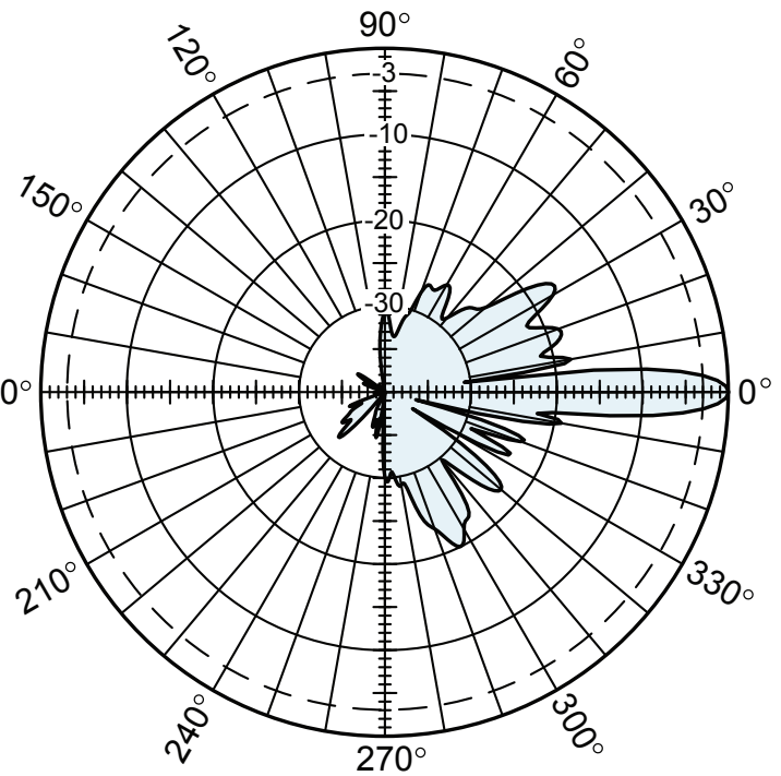
Antennekarakteristikk for en vanlig basestasjonsantenne for GSM900 mobiltelefoni
