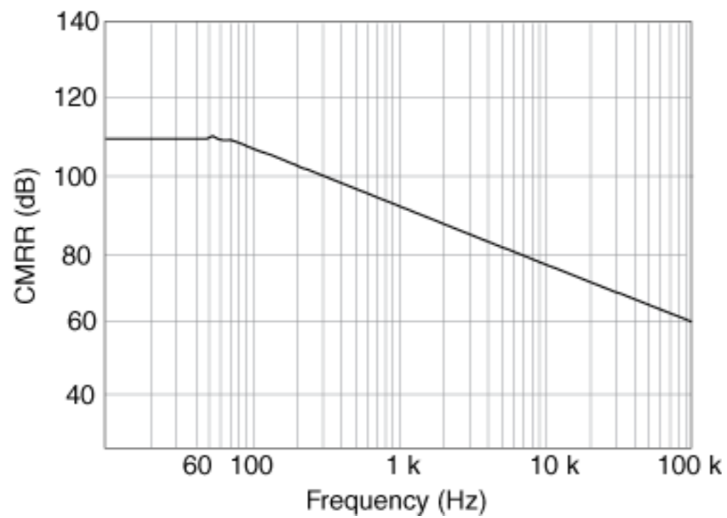
AI <0..31> CMRR
