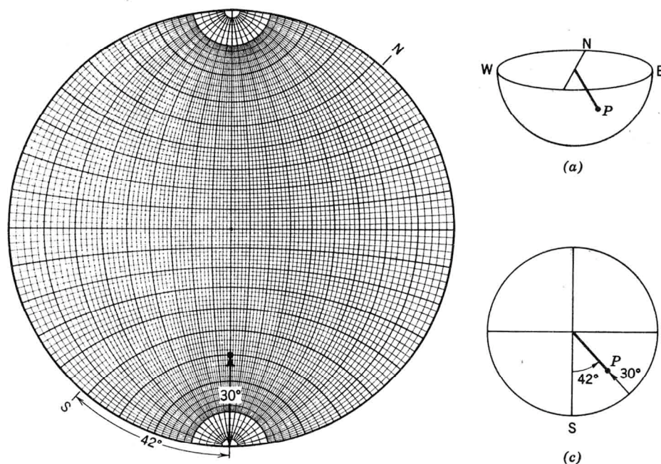
Fig.6: a): Perspektivisk bilde av linje (trend: N138°E; plunge: 30°E) b): Plotting av linjestrukturen på stereonettet. c): Stereografisk projeksjon av linjestrukturen. (Merk: projeksjonen er kun punktet (P))
