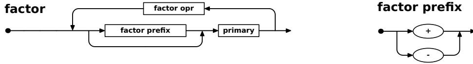
Figur 2.18: Jernbanediagram for \langle \text{factor} \rangle og \langle \text{factor prefix} \rangle
