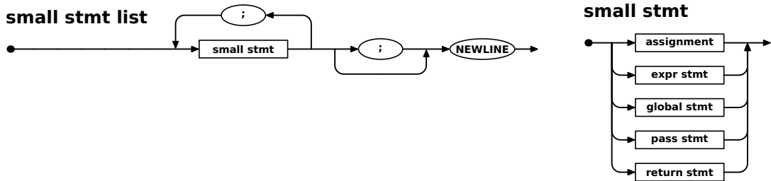
Figur 2.4: Jernbanediagram for <small stmt list> og <small stmt>
