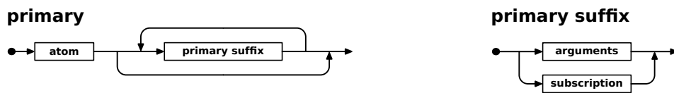
Figur 2.20: Jernbanediagram for \langle \text{primary} \rangle og \langle \text{primary suffix} \rangle
