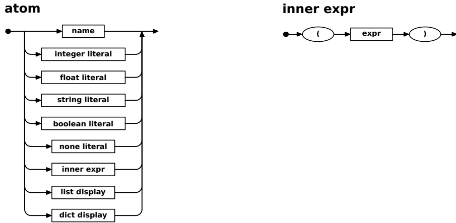
Figur 2.21: Jernbanediagram for ⟨atom⟩ og ⟨inner expr⟩
