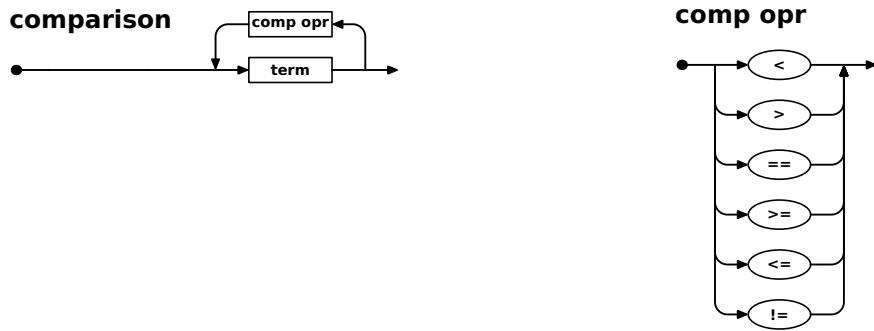
Figur 2.16: Jernbanediagram for \langle \text{comparison} \rangle og \langle \text{comp opr} \rangle
