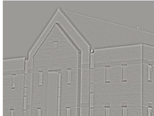
LoG-filtrering
