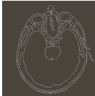
Cannys kantdetektor
