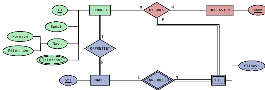
Figure 1: Løsningsforslag modellering
