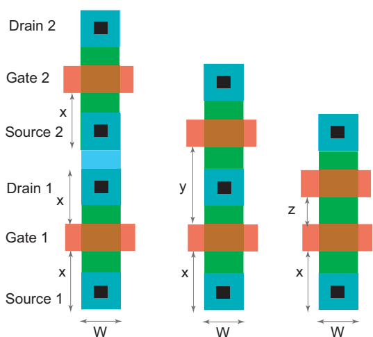
Fig. 3. Ulike geometrier for diffusjonsområder. (FIG2.8)
