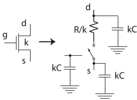
Fig. 9. Ekvivalent RC krets for en nMOS transistor med bredde lik k . (FIG3.5 øverst)
