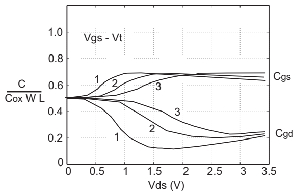
Fig. 5. Gate source- og gate drain kapasitanser.
