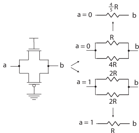
Fig. 13. Ekvivalent RC krets for transmisjonsport.
