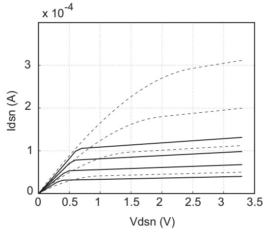
Fig. 19. I - V karakteristikk for lang og kort transistor med kanal-lengdemodulasjon.
