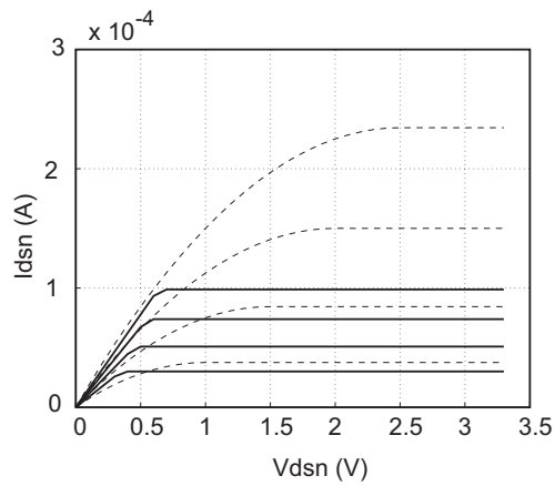
Fig. 18. I - V karakteristikk for lang og kort transistor med enkle modeller. (FIG2.16)
