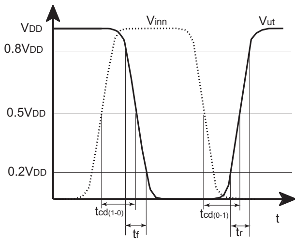
Fig. 14. Definisjon av tidsforsinkelser (FIG3.1).
