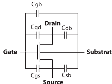
Fig. 8. Kapasitanser knyttet til en nMOS transistor. (FIG2.13)
