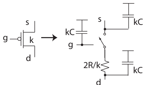
Fig. 10. Ekvivalent RC krets for en pMOS transistor med bredde lik k . (FIG3.5 nederst)
