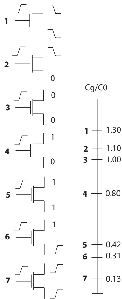
Fig. 6. Gate kapasitans for ulike signalnivåer og signaltransisjoner på source og drain.(FIG2.11)
