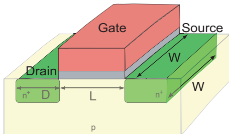
Fig. 7. Geometrier for diffusjonsområder. (FIG2.12)
