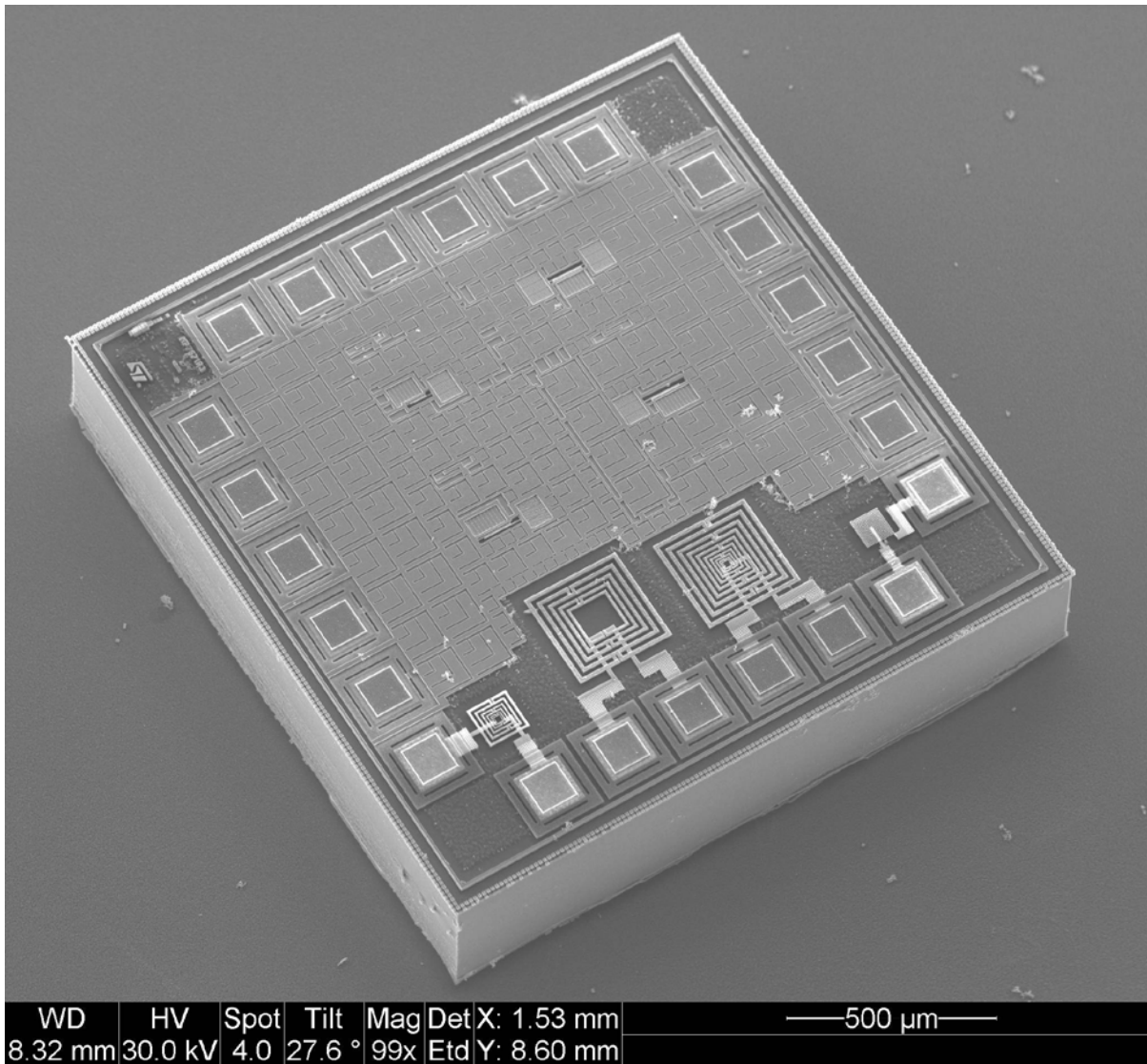
IFI test circuits from STM (JER, JE)
