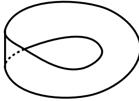
Fig. 21.5. Möbius band.
